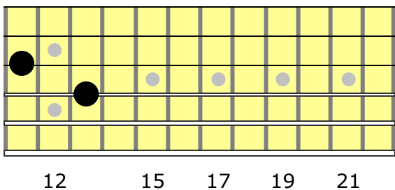
D#m
