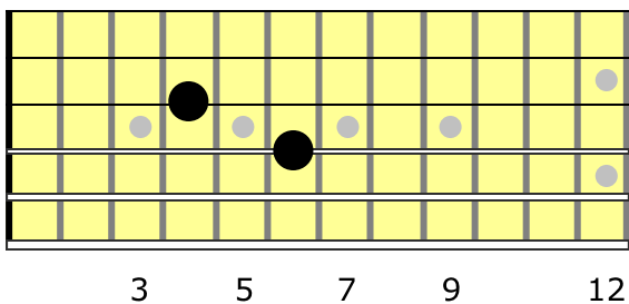
G#m
