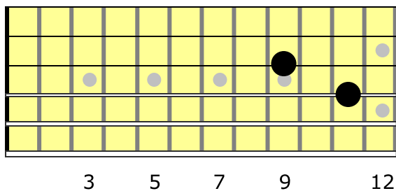
C#m
